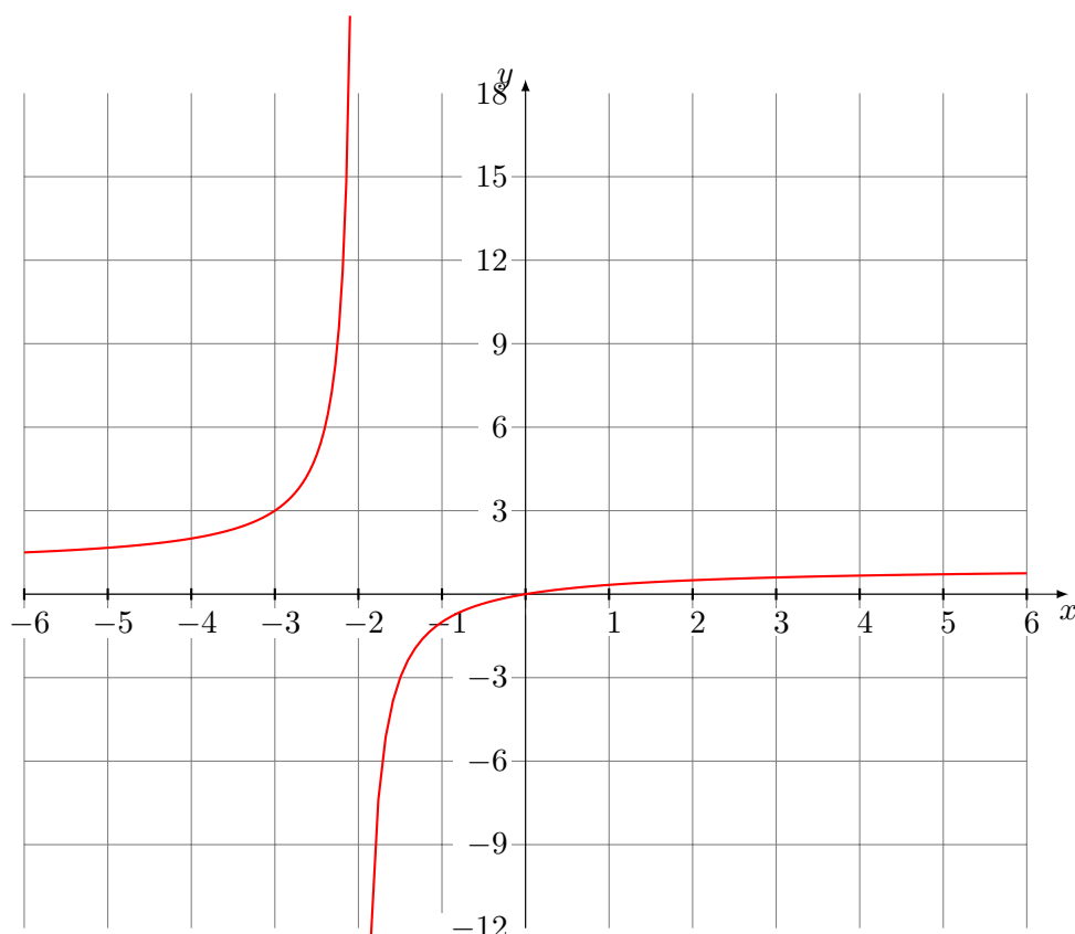
Figure 14: Representación de la función f(x) = \frac{x}{x+2}
