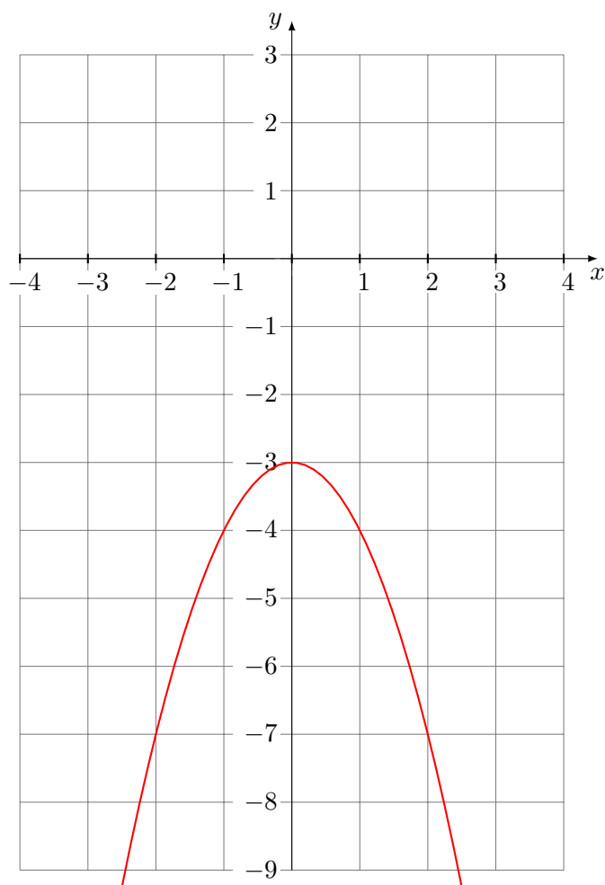
Figure 3: Representación de la función f(x) = -x^2 - 3
