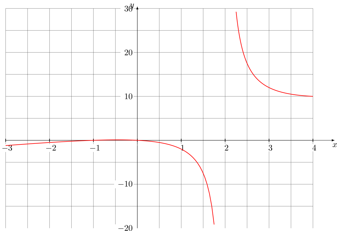
Figure 15: Representación de la función f(x) = \frac{x(x+1)}{x-2}
